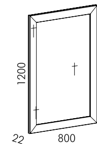
Зеркало 800x1200 (возможна вертикальная и горизонтальная навеска)
